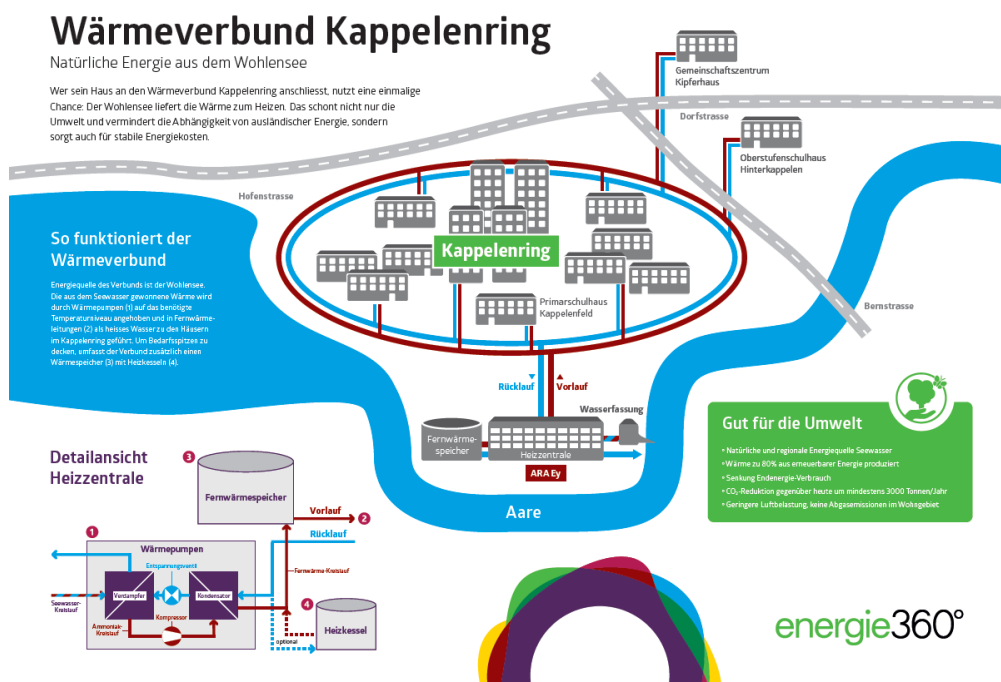
Das Schema zeigt die Funktionsweise des Wärmeverbunds auf.
